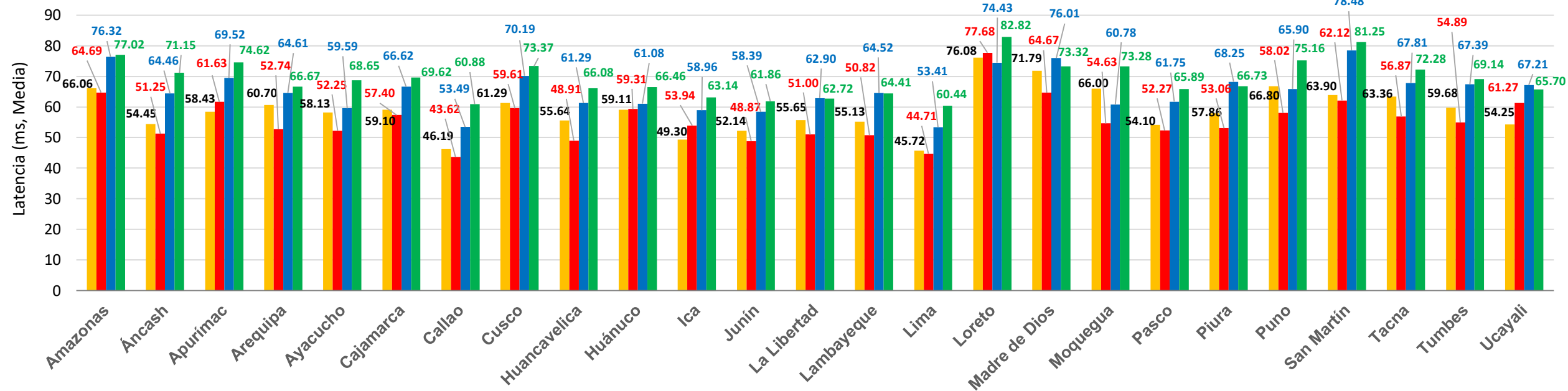
Latencia promedio 4G a nivel nacional
