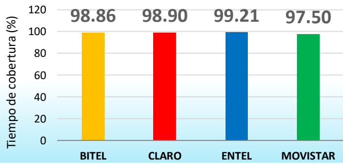
Tiempo de cobertura 3G+4G+5G a nivel nacional
