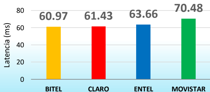
Latencia promedio 3G+4G+5G a nivel nacional
