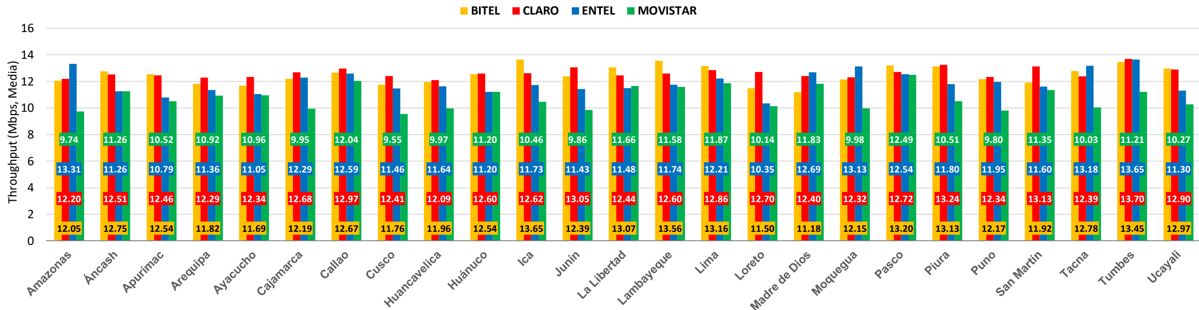
Velocidad promedio descarga 4G a nivel nacional
