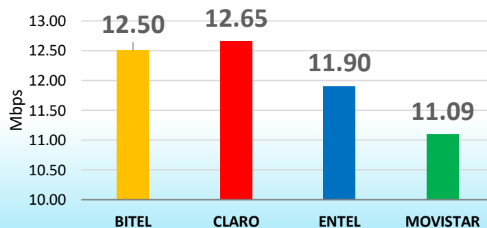
Velocidad promedio descarga 4G a nivel nacional
