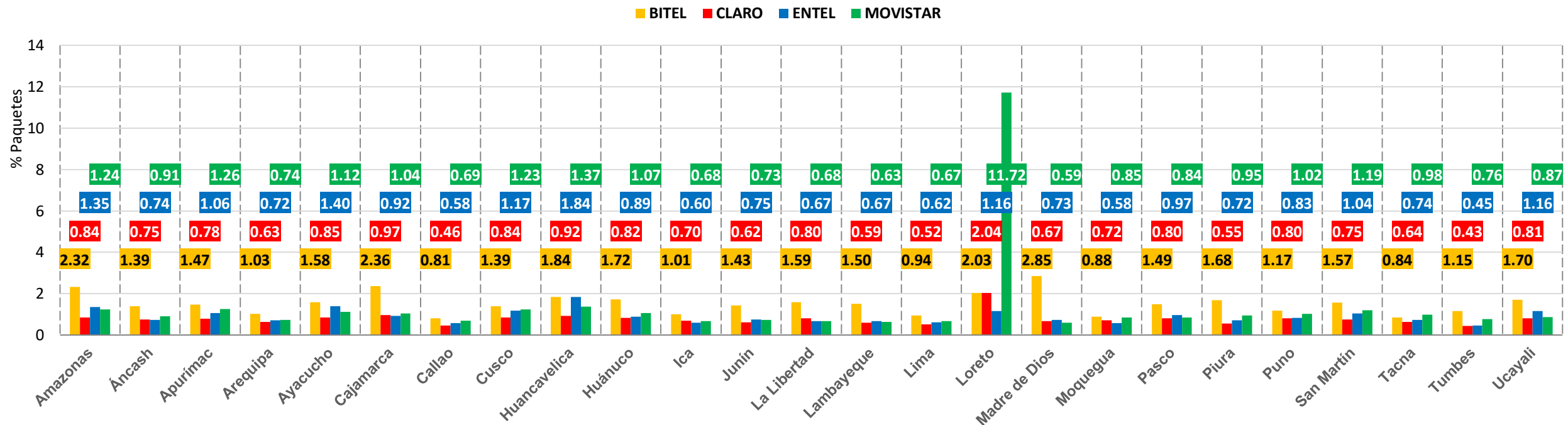
Pérdida de paquetes 3G+4G+5G a nivel nacional
